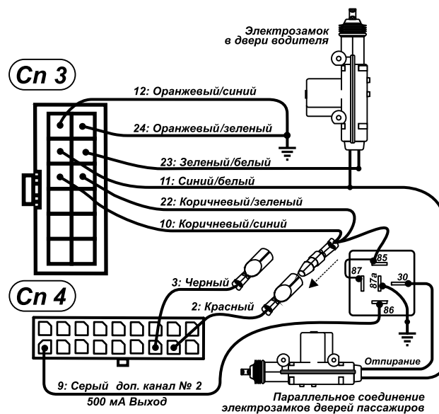
Схема приоритетного отпирания двери водителя
