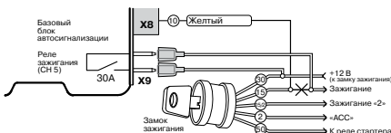
Типовая схема подключения к замку зажигания (с разрывом)
