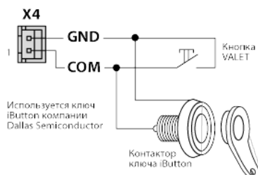
Подключение контактора ключа iButton
