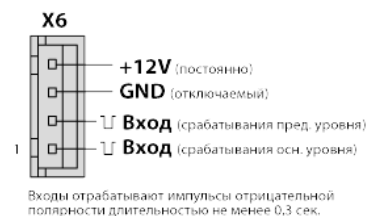
Подключение дополнительного датчика
