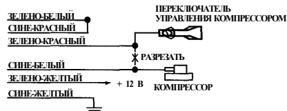
СХЕМА С ПНЕВМАТИЧЕСКИМ УПРАВЛЕНИЕМ ЗАМКАМИ
