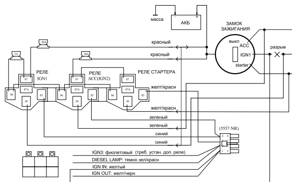
СХЕМА СОЕДИНЕНИЙ В РЕЖИМЕ АВТОЗАПУСКА БЕЗ ИСПОЛЬЗОВАНИЯ ДОПОЛНИТЕЛЬНОЙ ЦЕПИ IGN OUT
