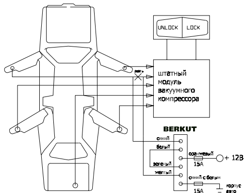
СХЕМА УПРАВЛЕНИЯ ВАКУУМНЫМИ СИСТЕМАМИ Mercedes-Banz, Audi
