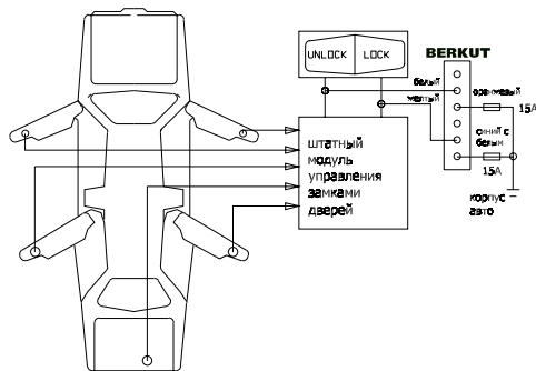
Отрицательный триггер (большинство автомобилей японского производства)
