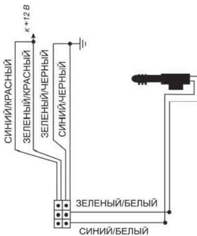
Схема 6. Установка дополнительных электропроводов
